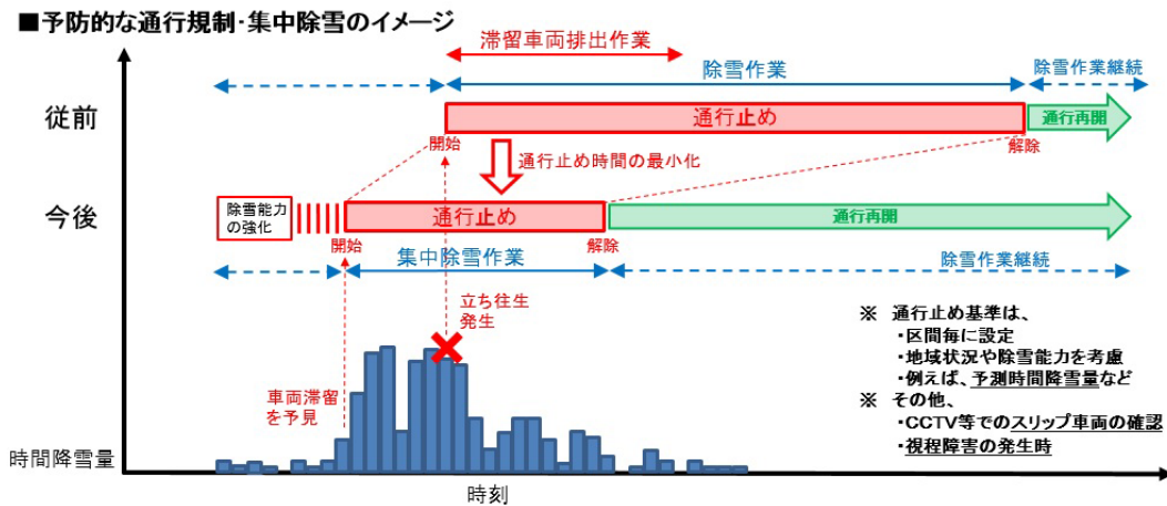
図7 予防的な通行規制・集中除雪のイメージ
