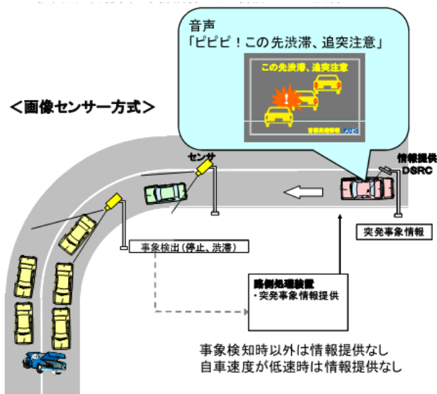
図4-1 渋滞末尾情報の概要（赤外線カメラ方式）
