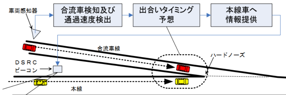
図 4 - 3 合流支援サービスの基本枠組み
