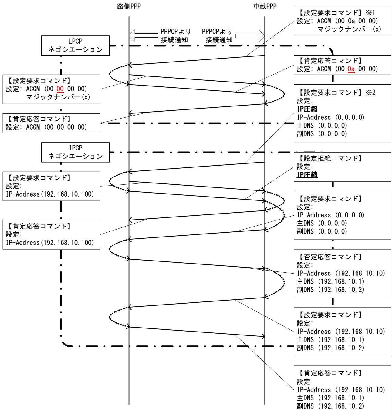
図 4-2 PPP ネゴシエーションシーケンス例 2
